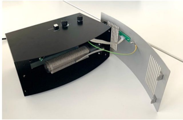
Abb. 3 und 4: Gerätemontage
